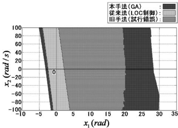
図 - 5 安定領域の比較
