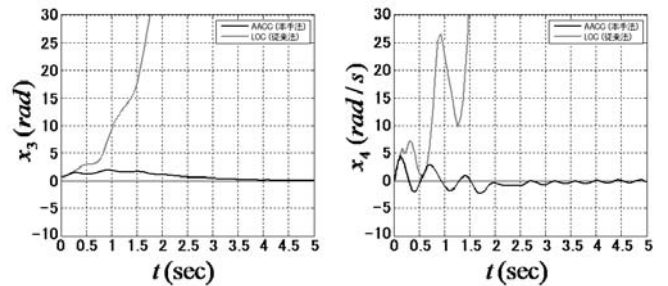
図 - 7 x_3, x_4 (種子島第一: 10号機) の時間応答
