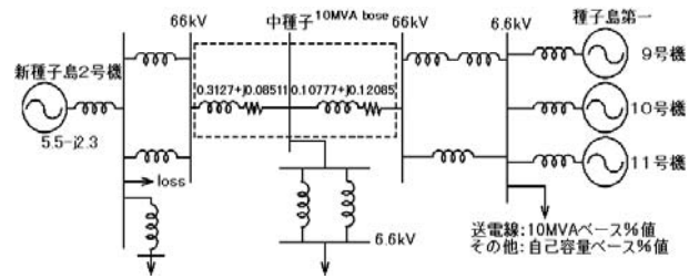
図 - 3 種子島電力系統図
