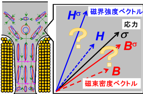
図1：実機モータの磁気現象
