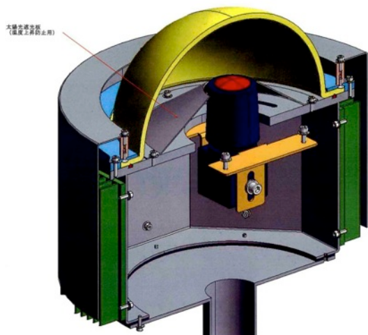
図1：設計したカメラハウジングの断面図
