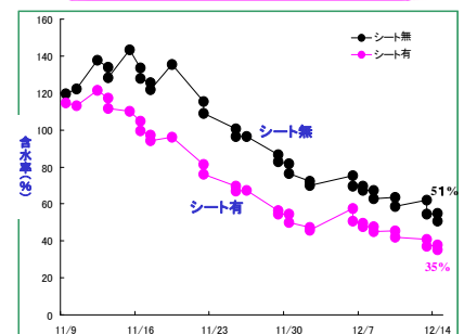
シート被覆の有無による含水率減少の経過
