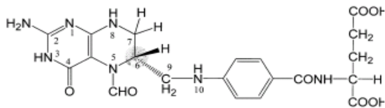
図 2. LV の構造
