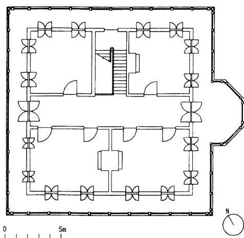
図-13 異人館2階復元平面図 2)
