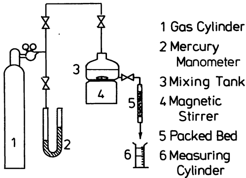
図1 分離装置の概略
