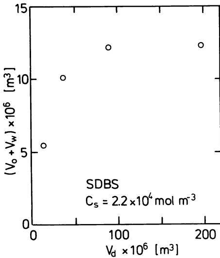
図7 アルミナの再生における水量と分離流出量との関係
