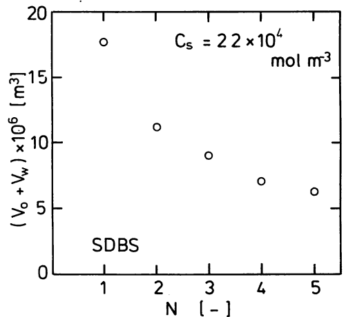
図8 再生回数と分離流出量との関係
