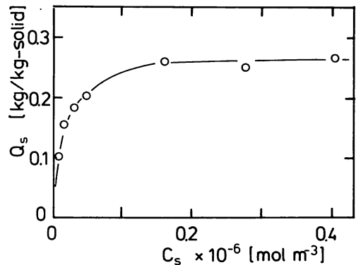
図6 SDBS のアルミナに対する吸着 (297 K)
