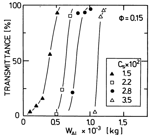
図10 エマルジョンの分離に対するアルミナ添加の効果 (界面活性剤がオレイン酸Mgの場合)
