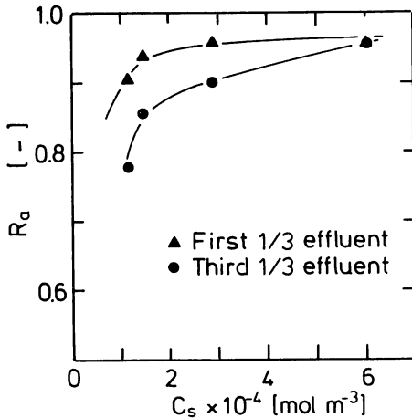
図5 エマルション中の SDBS がアルミナに吸着される割合
