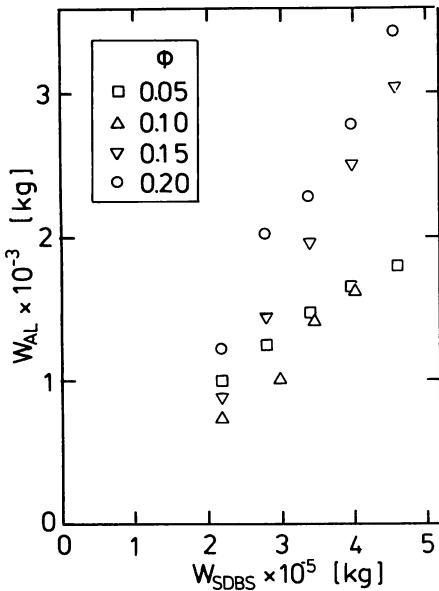
図11 分離に必要なアルミナ量に対する SDBS 濃度の影響
