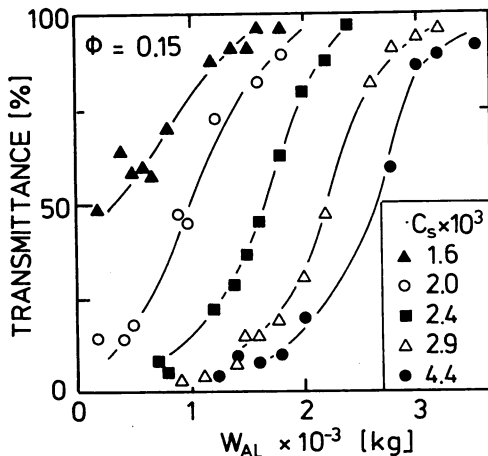
図9 エマルジョンの分離に対するアルミナ添加の効果 (界面活性剤がSDBSの場合)
