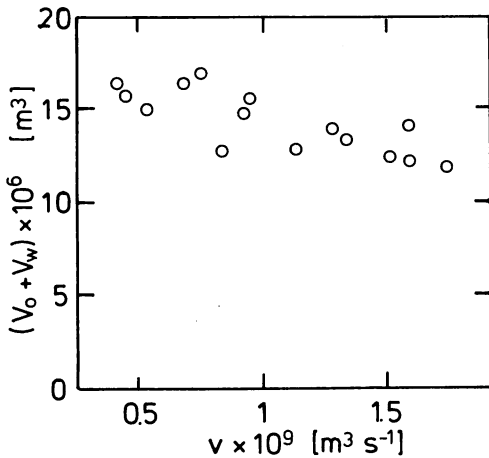
図3 分離流出量と流出速度との関係
