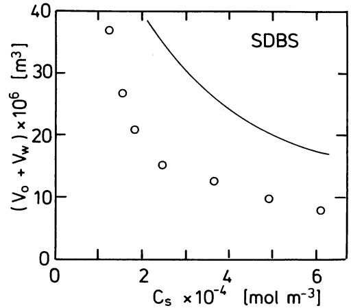
図4 破過するまでの分離流出量に対する SDBS 濃度の影響 (実線は計算による予測値)
