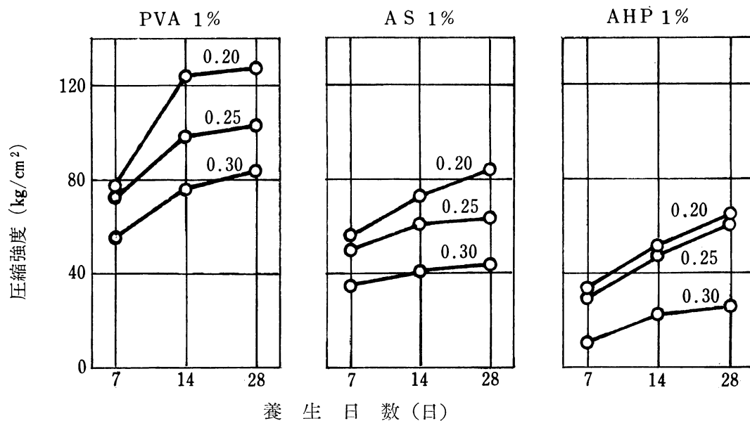
図 2 シラス-石灰モルタルにおよぼす水/粉比の影響
