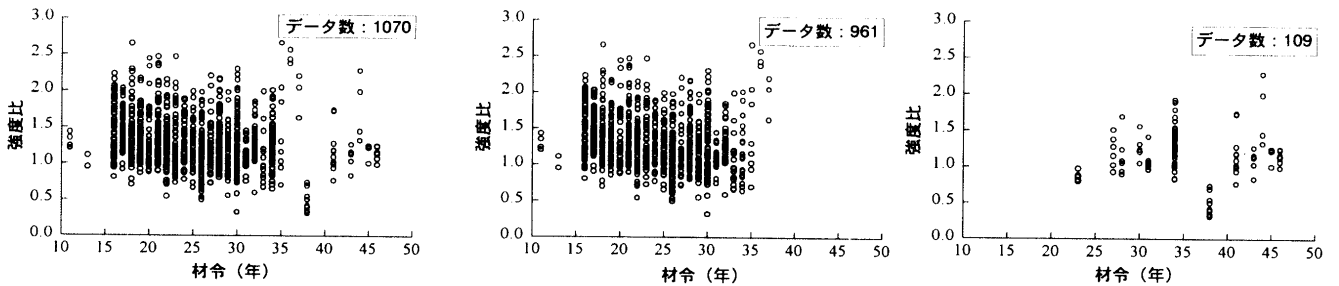
図10 強度比と材令の関係
