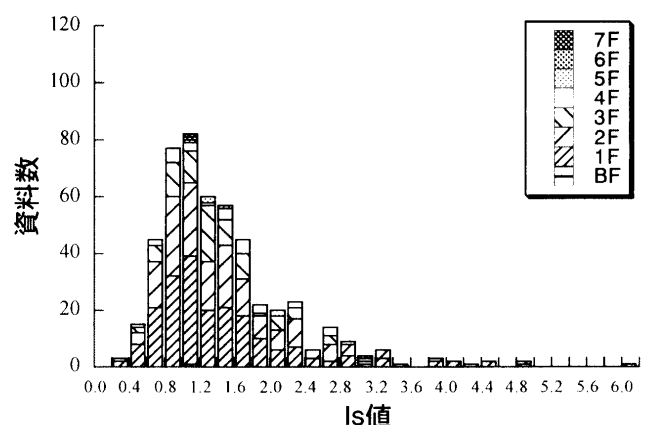
図3 Y方向の階別のIs値
