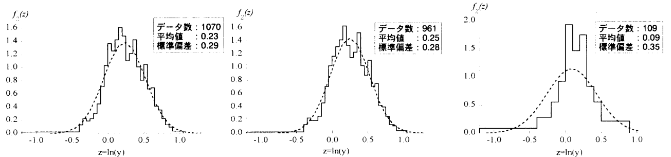
図8 Z=ln(Y)の分布
