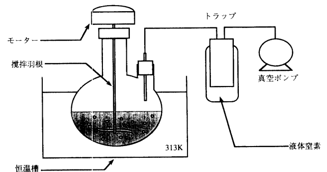
Fig.1 装置図
