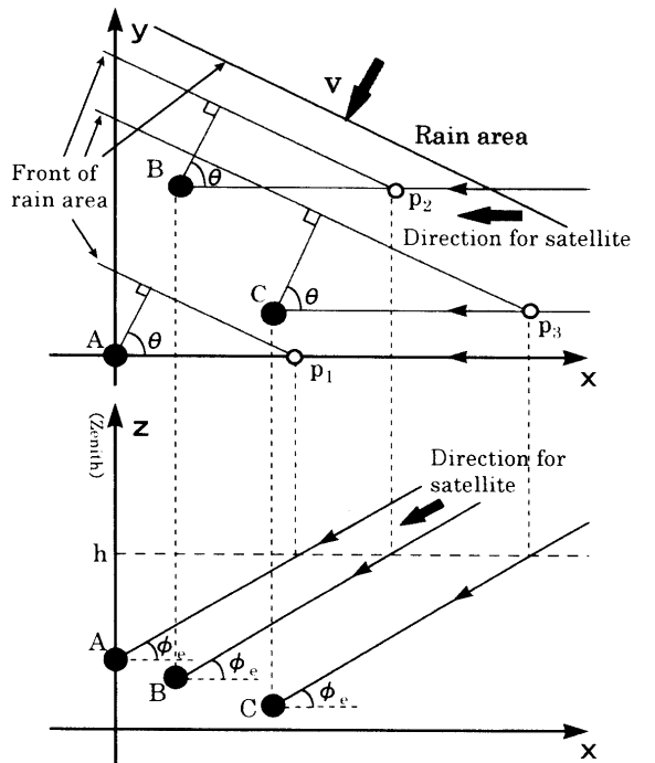
A, B, C: 観測局 \phi_e : 衛星仰角 A局点座標: (0, 0, z_1) h : 雨域の高さ B局点座標: (x_2, y_2, z_2) v : 雨域移動速度 C局点座標: (x_3, y_3, z_3) \theta : 雨域移動方向の x 軸に対する角度 P_1 : 雨域前面のA局点衛星電波通路進入地点 P_2 : 雨域前面のB局点衛星電波通路進入地点 P_3 : 雨域前面のC局点衛星電波通路進入地点
