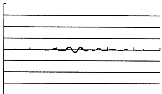
図10 水とのマッチングを意図して作られた商用設計のフェライトゴムの、水との界面の反射波
