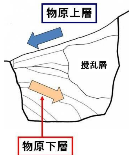
物原トレンチ南壁断面図
