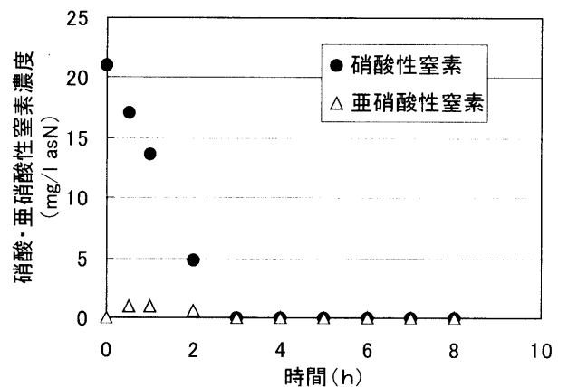
図5 アルギン酸カルシウムビーズ 3g(wet 質量)を用いた脱窒実験結果
