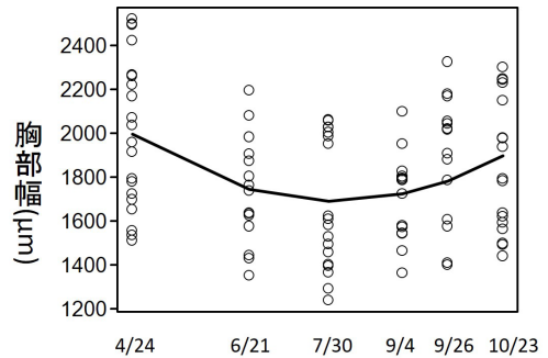
図 4. ヤマトシジミの体サイズの季節変化。曲線は二次の多項式回帰を当てはめたもの。
