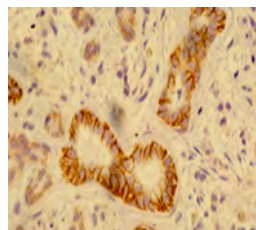
図-5 Na/K-ATPase
