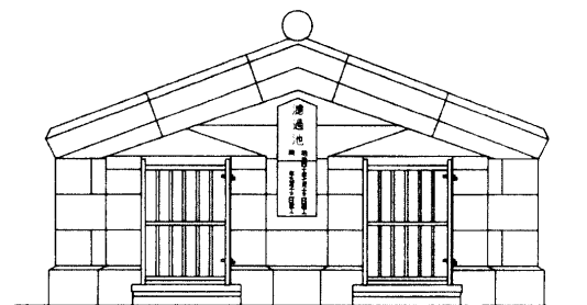
図一8 家形石造ろ過池覆屋正面図
