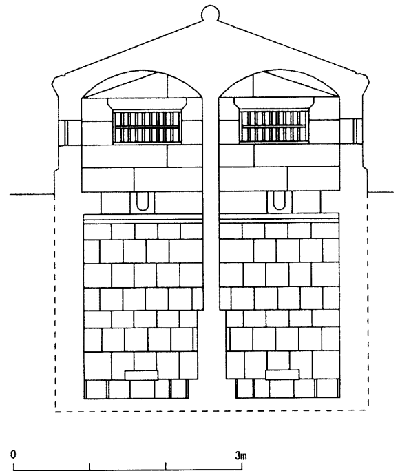
図一6 家形石造ろ過池覆屋横断面図
