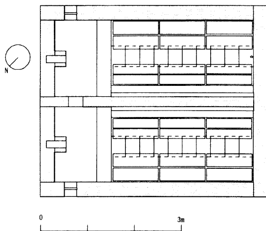
図一5 家形石造ろ過池覆屋平面図
