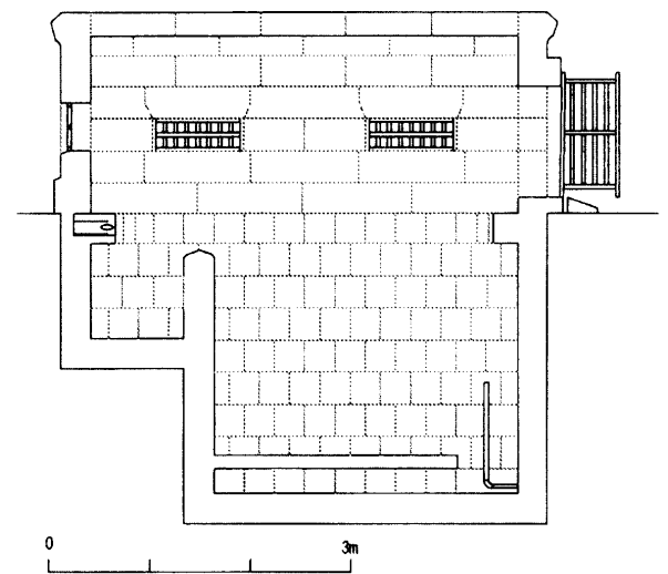
図一7 家形石造ろ過池覆屋縦断面図
