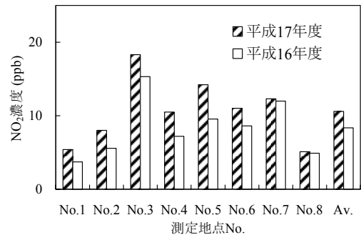
図-13 測定地点別年平均NO 2 濃度
