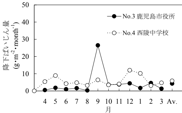
図-4 測定地点別降下ばいじん量
