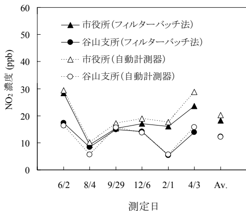
図-15 フィルターバッチ法と自動計測器による NO 2 濃度
