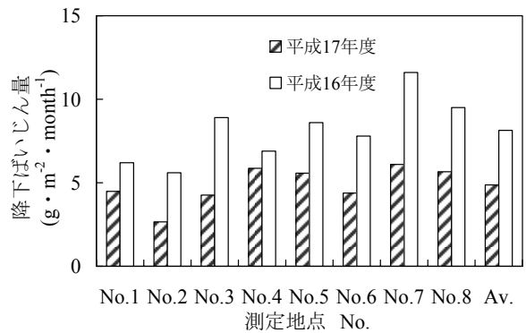
図-7 測定地点別年平均降下ばいじん量
