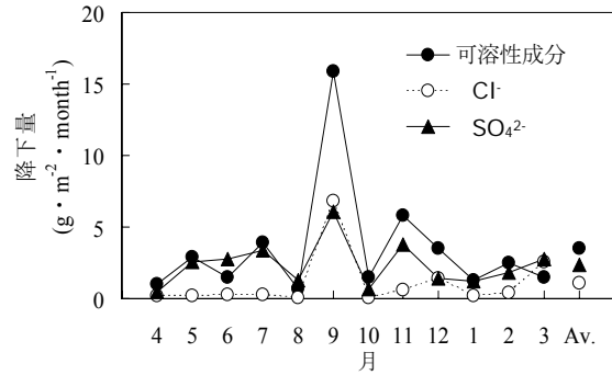
図-11 8地点平均可溶性成分、SO 4 2- 、Cl - 降下量
