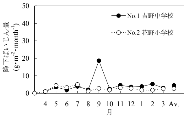
図-3 測定地点別降下ばいじん量
