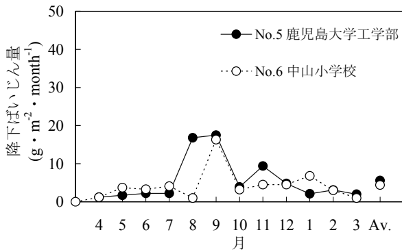
図-5 測定地点別降下ばいじん量
