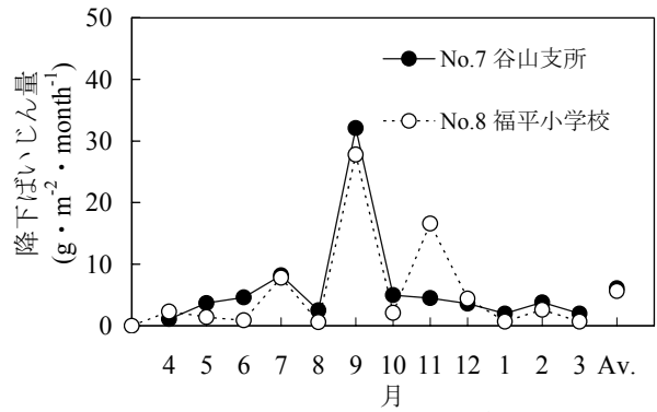
図-6 測定地点別降下ばいじん量
