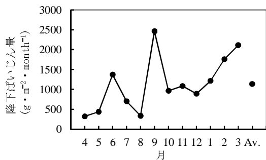
図-10 桜島 14 地点平均降下ばいじん量
