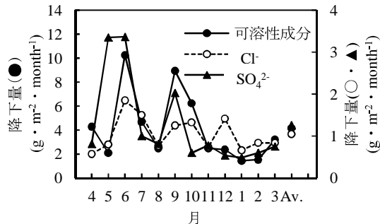
図-11 8 地点平均可溶性成分、SO 4 2- 、Cl - 降下量
