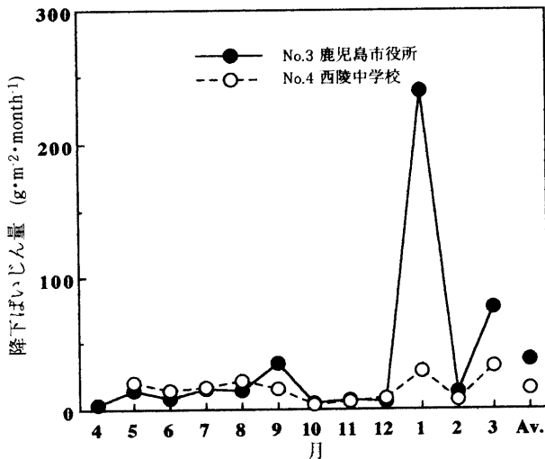
図4 No.3 鹿児島市役所, No.4 西陵中学校における月別降下ばいじん量
