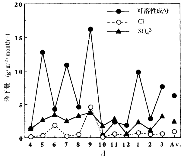
図11 8測定地点平均月別可溶性成分、SO₄²⁻、Cl⁻ 降下量
