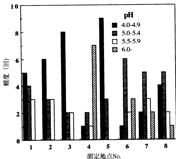
図12 測定地点別のpH段階別頻度
