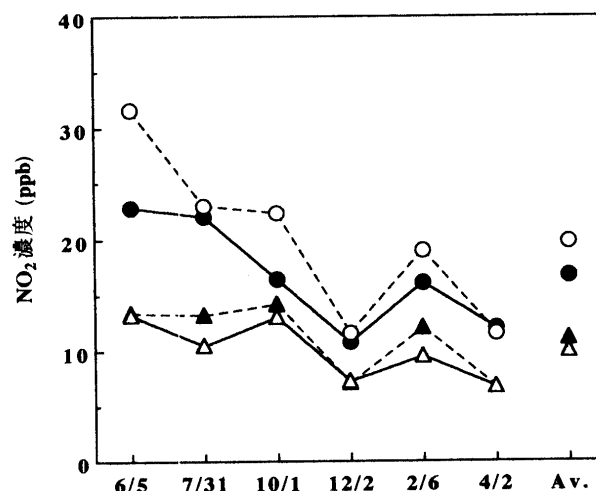
図15 フィルターバッジ法と自動計測器によるNO 2 濃度
