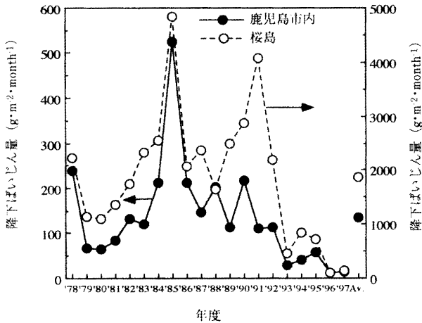
図8 鹿児島市内平均および桜島全島平均年度別降下ばいじん量
