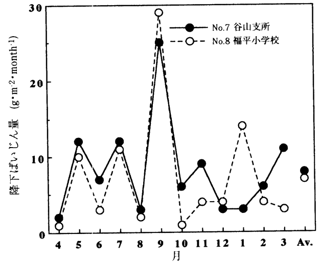
図6 No.7 谷山支所, No.8 福平小学校における月別降下ばいじん量
