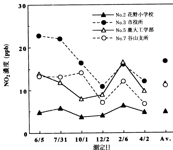
図14 4測定地点におけるNO 2 濃度
