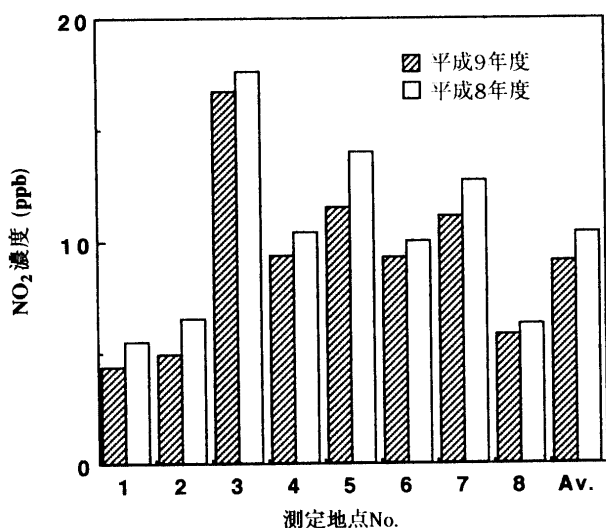
図13 測定地点別年平均NO 2 濃度
