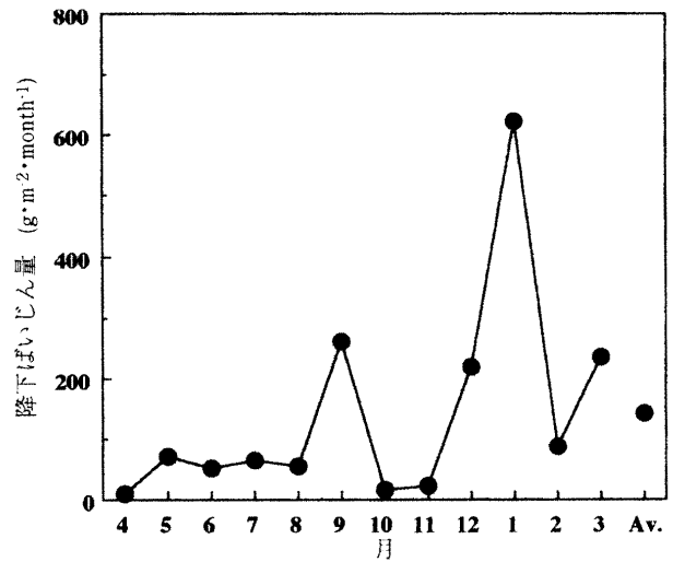
図10 桜島14地点平均月別降下ばいじん量
