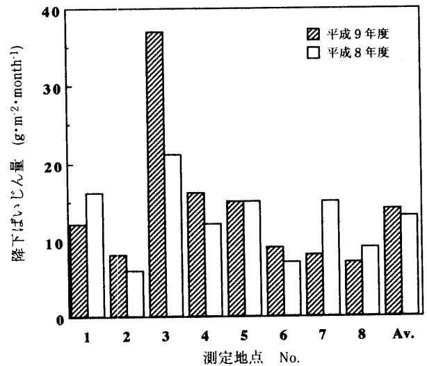
図7 測定地点別年平均降下ばいじん量
