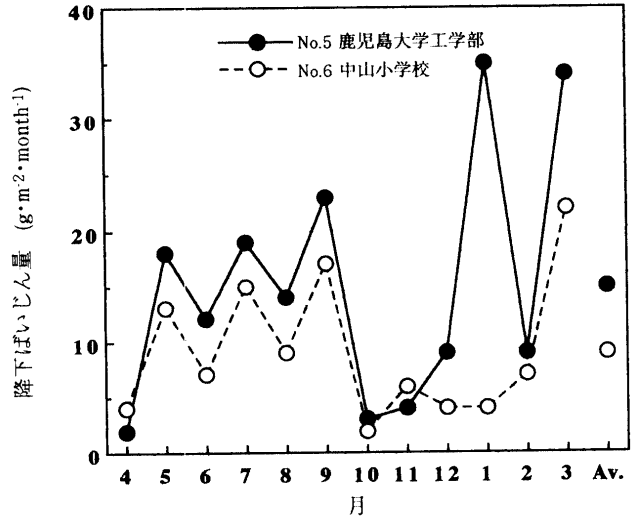
図5 No.5 鹿大工学部, No.6 中山小学校における月別降下ばいじん量
