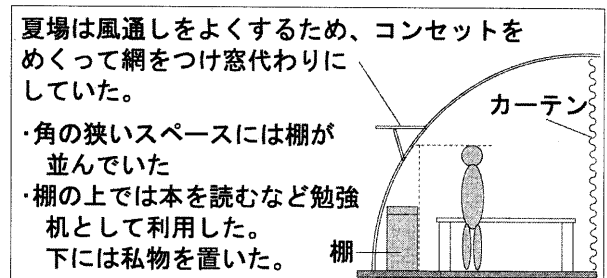
図-8 コンセット断面図
