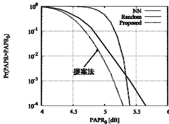
図 3. ピーク電力抑圧性能(左側に位置するほど抑圧性能は高い)
