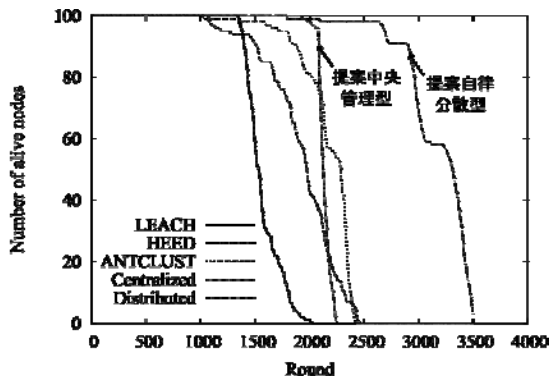
図 1. ノード密度が低い場合のラウンド数に対する稼働ノード数の変化
