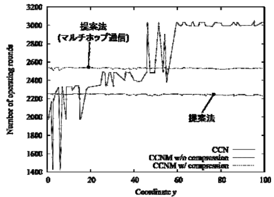
図 2. 基地局からの距離に対する各ノードの稼働ラウンド数
