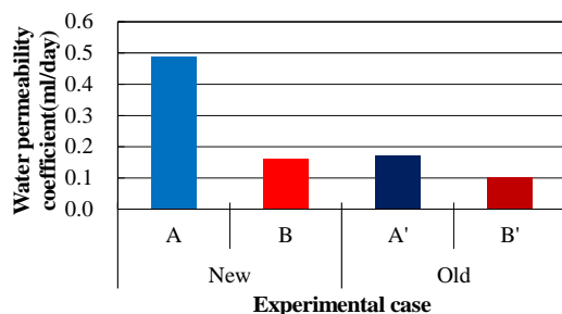
図-4 透水量試験
