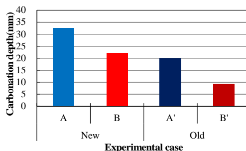
図-6 中性化試験
