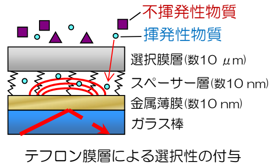
醸造酒のアルコール度数測定
