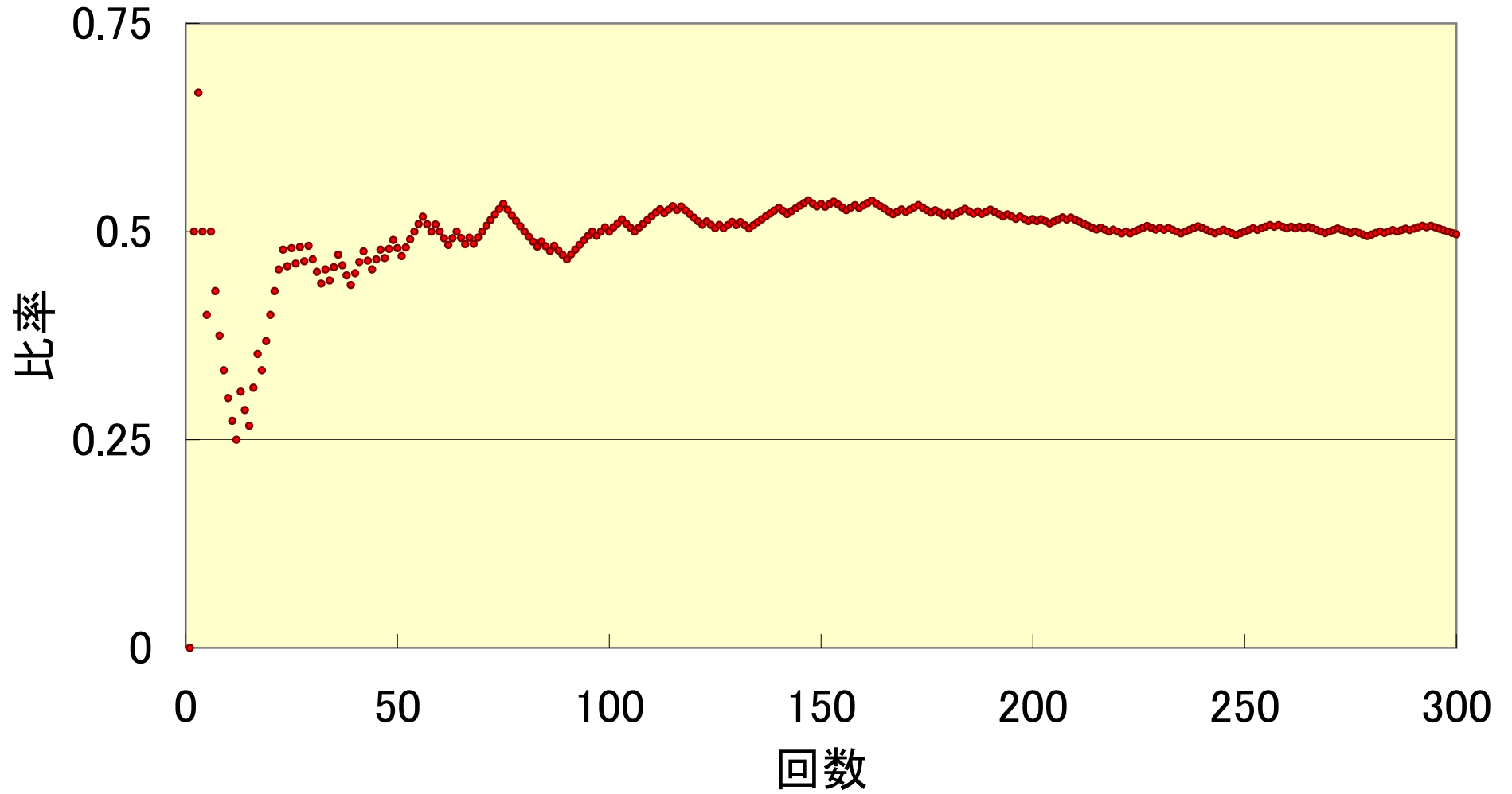
模擬貨幣投げ表の比率：表を確率0.5で
