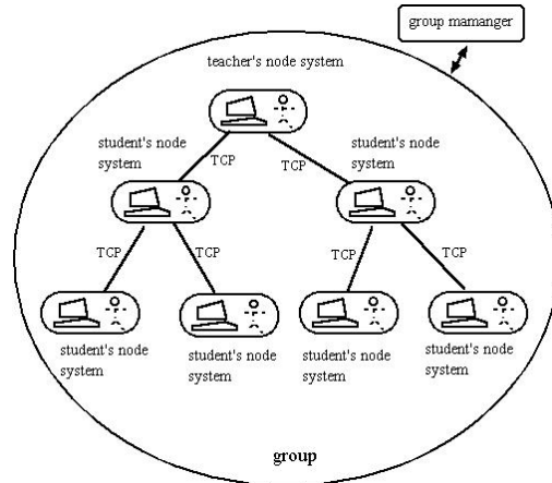
図 1. SOLAR-CATS の構成
